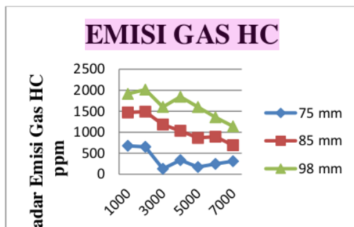
Gambar 3.2 Grafik Emisi Gas HC
