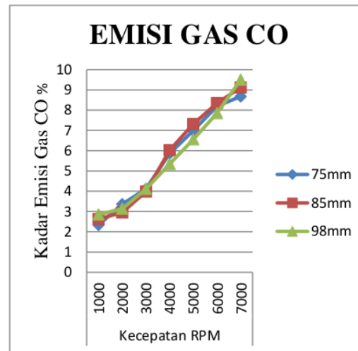
Gambar 3.1 Grafik Emisi Gas CO
